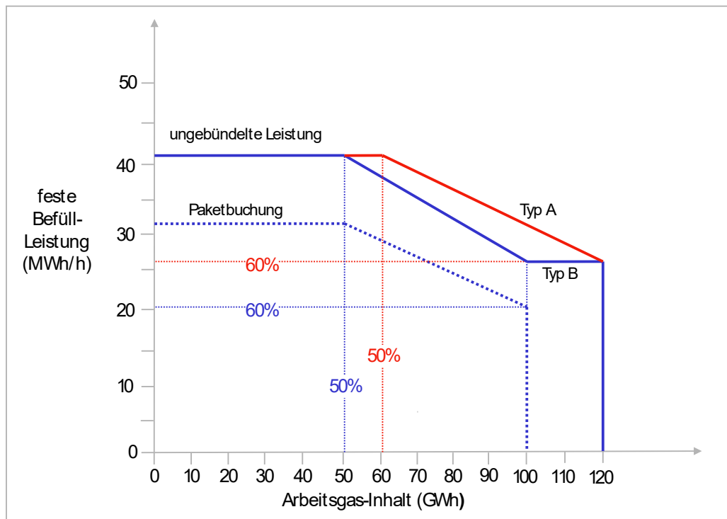
Abbildung 2: Kennlinie Befüllleistung bei fester Speicherkapazität
