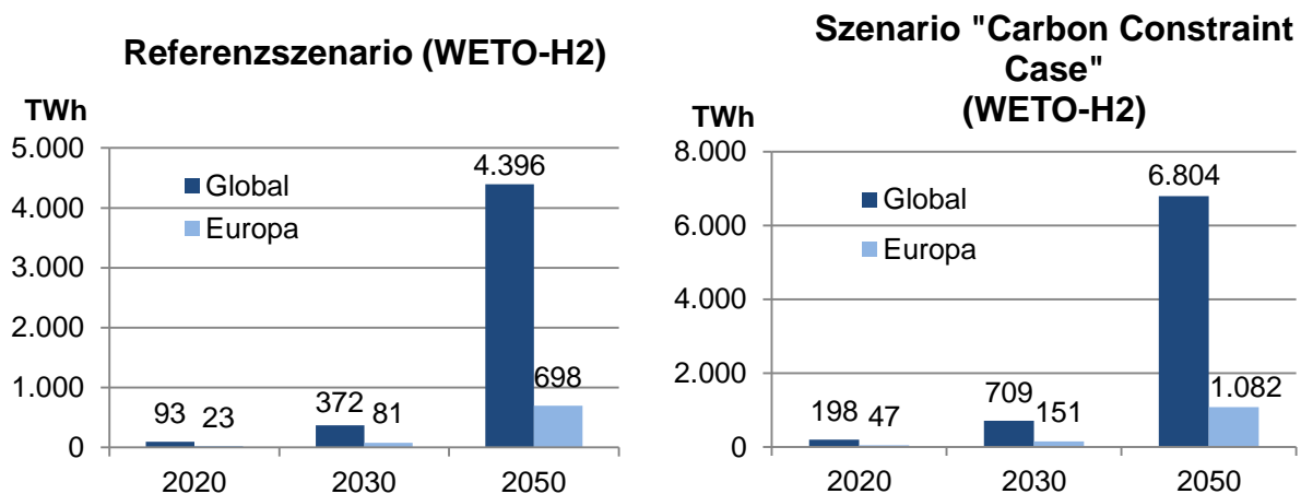
Abbildung 2: Prognostizierte energetisch bedingte zusätzliche Entwicklung der Wasserstoffproduktion (Quelle: EU-Kommission (2006))
