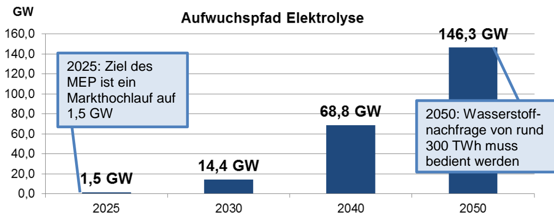
Abbildung 1: Aufwuchspfad der zu installierenden Elektrolysekapazitäten in Deutschland (kumuliert)
